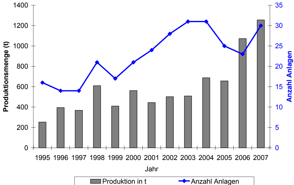
Abb. 8: Entwicklung der Produktionsmenge (graue Säulen) sowie der Anzahl gemeldeter Kreislaufanlagen (blaue Linie) im Zeitraum 1995-2007
