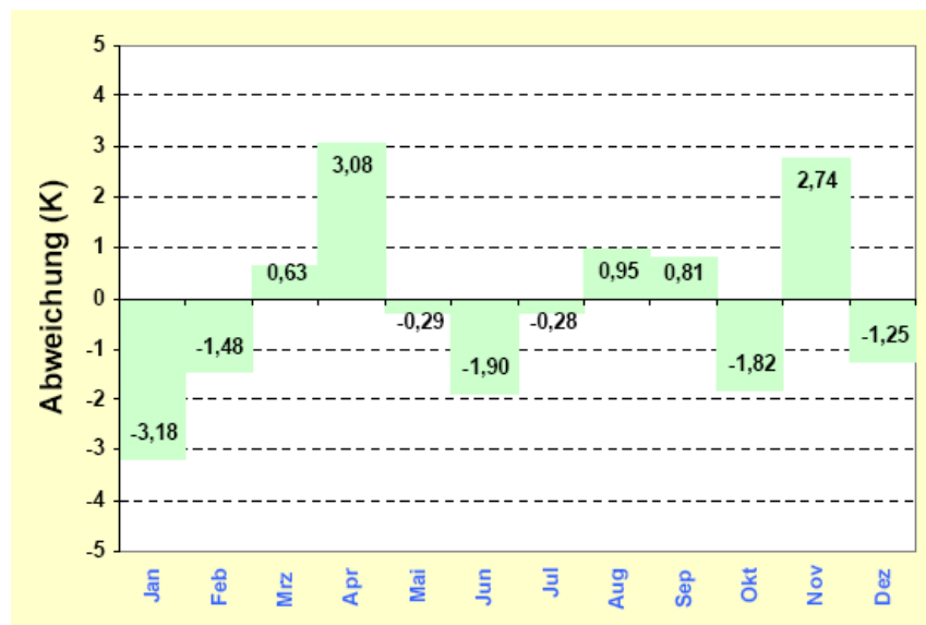
Abb. 7: Abweichungen der Tagesmittelwerte der Lufttemperatur 2009 in Königswartha vom langjährigen Mittel 6
